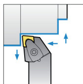
Rechtsausführung 95°
