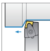
Rechtsausführung 75°
