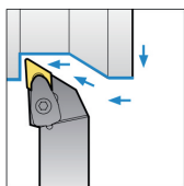
Rechtsausführung 93°
